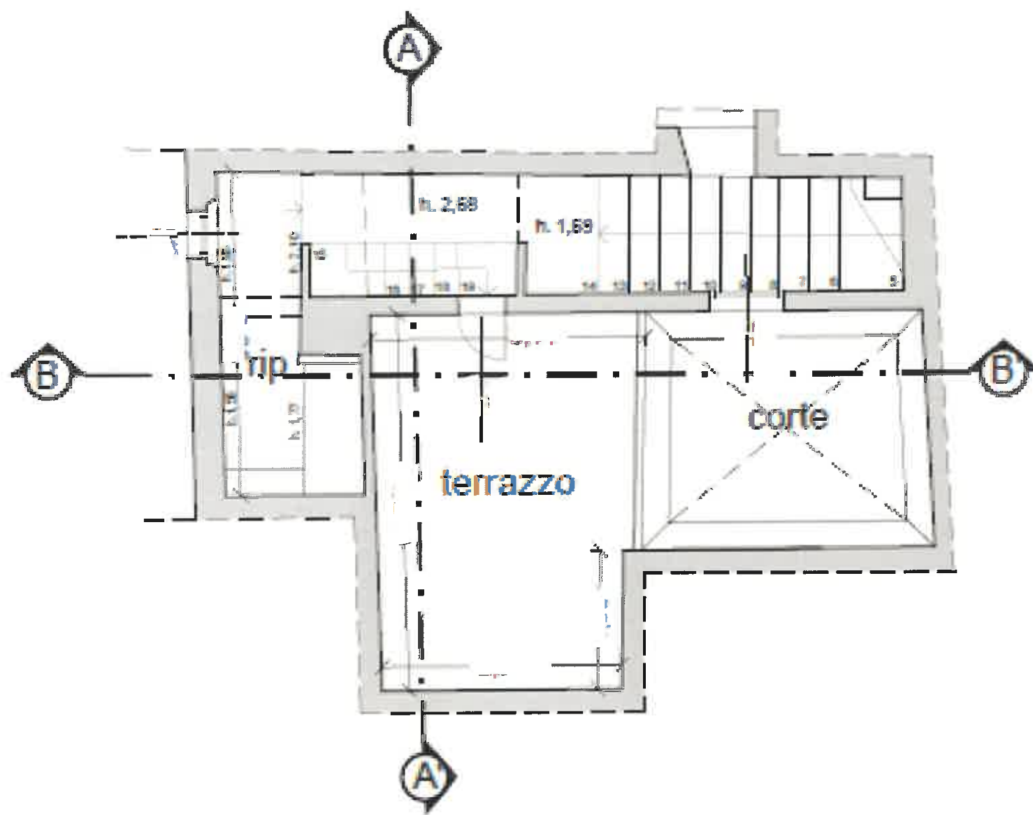
PIANTA PIANO QUARTO
